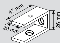
U-Trägertyp
