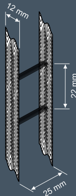
Leiterband 12 mm
