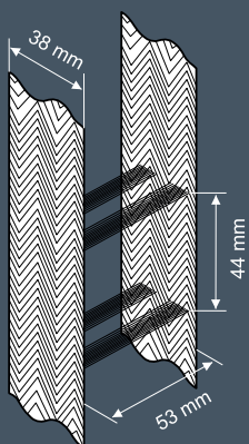
Leiterband 38 mm
